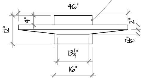
DÉTAIL TÉLÉVISEUR (bloc à faire)
