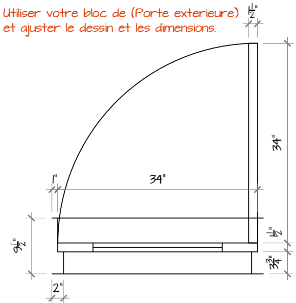
DÉTAIL PORTE EXTÉRIEURE
