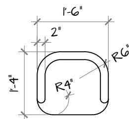
DÉTAIL CHAISE (bloc à faire)
